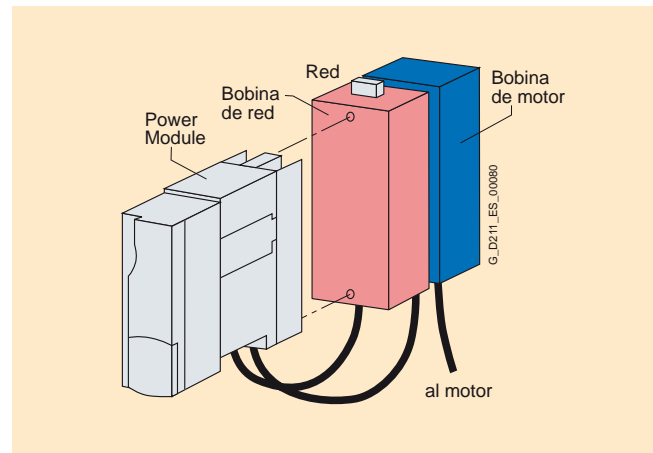
Power Module PM240 de tamaño FSA con bobina de red y bobina de motor
