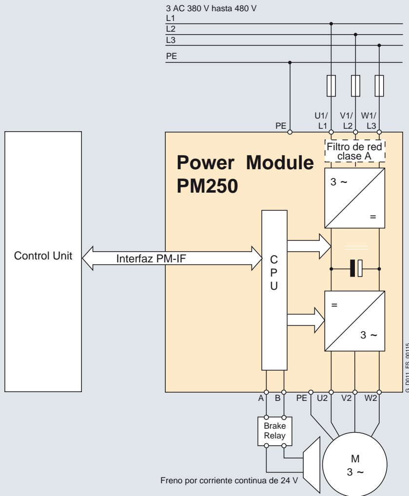
Esquema de conexiones Power Module PM250 con filtro de red de clase A integrado
