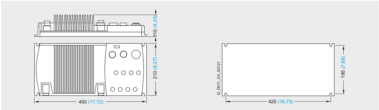
Power Module PM250D tamaño FSA con filtro de red de clase A integrado y Control Unit enchufada
