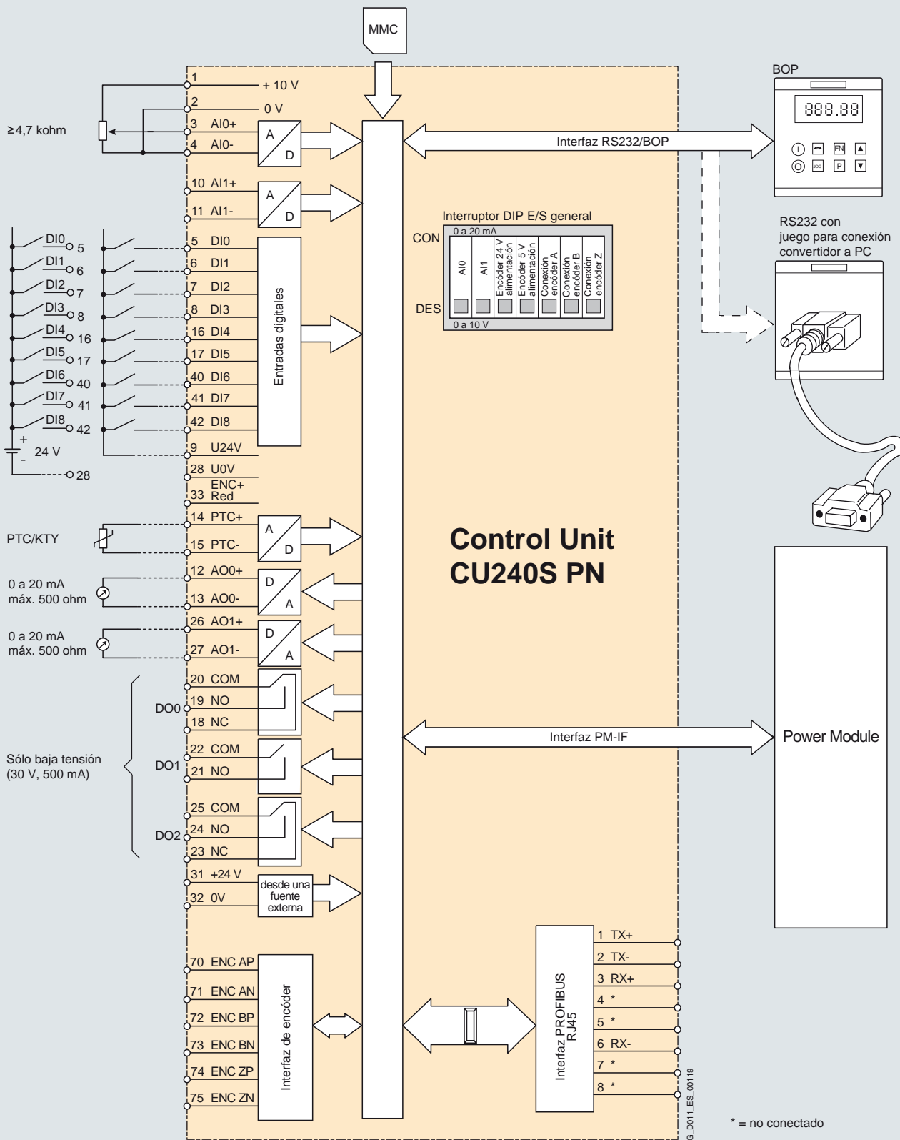
Esquema de conexiones Control Unit CU240S PN
