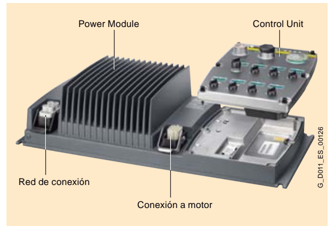
Power Module PM250D con conexión de red y del motor y Control Unit CU240D
