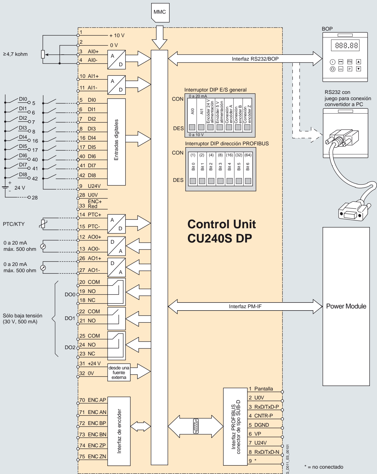
Esquema de conexiones Control Unit CU240S DP
