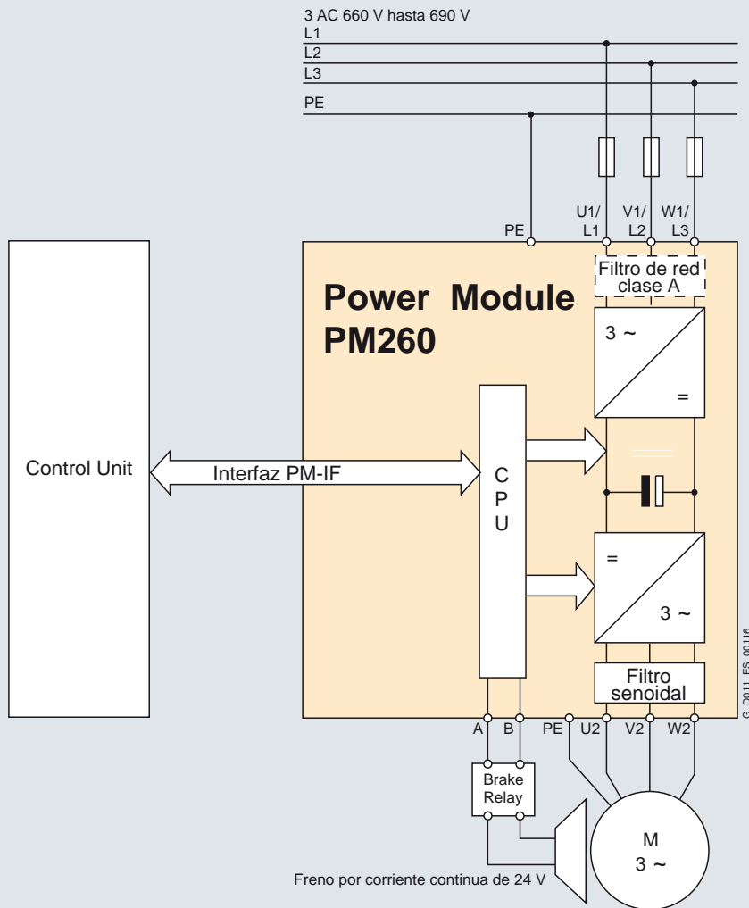
Diagrama de conexiones del Power Module PM260 con y sin filtro de red de clase A integrado
