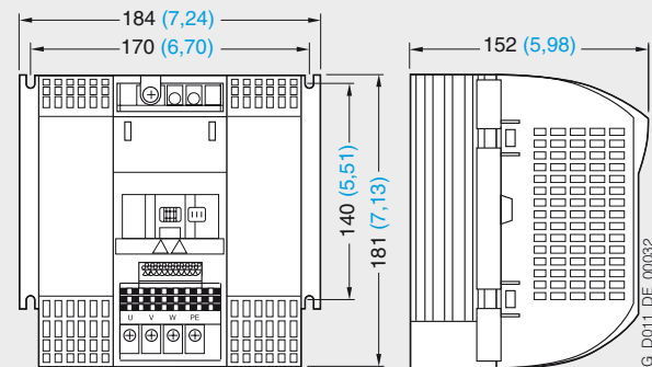
Convertidores FSC; 2,2 kW a 3,0 kW
