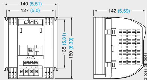
Convertidores FSB; 1,1 kW a 1,5 kW
