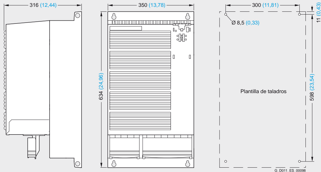
Power Module PM240 de tamaño FSF sin filtro de red
