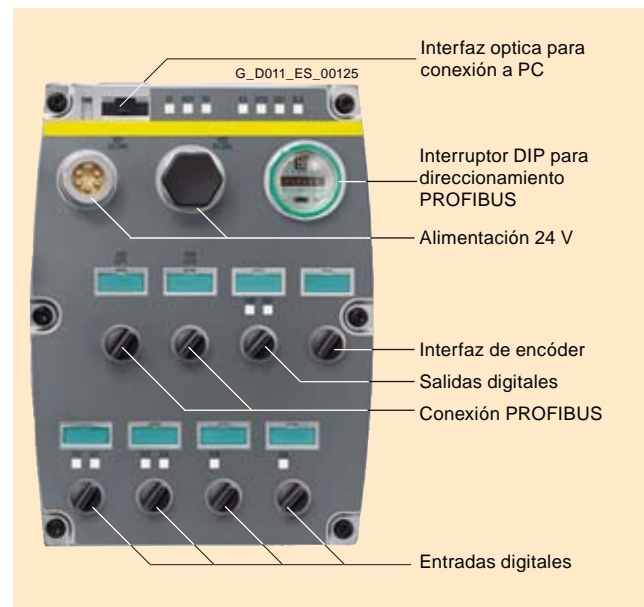
Conexiones Control Unit CU240D DP-F
