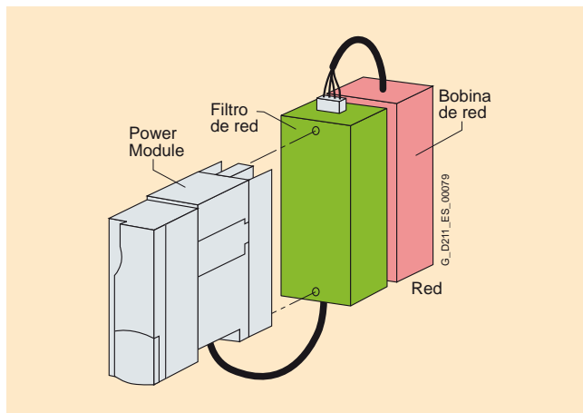
Power Module PM240 de tamaño FSA con bobina de red y filtro de red
