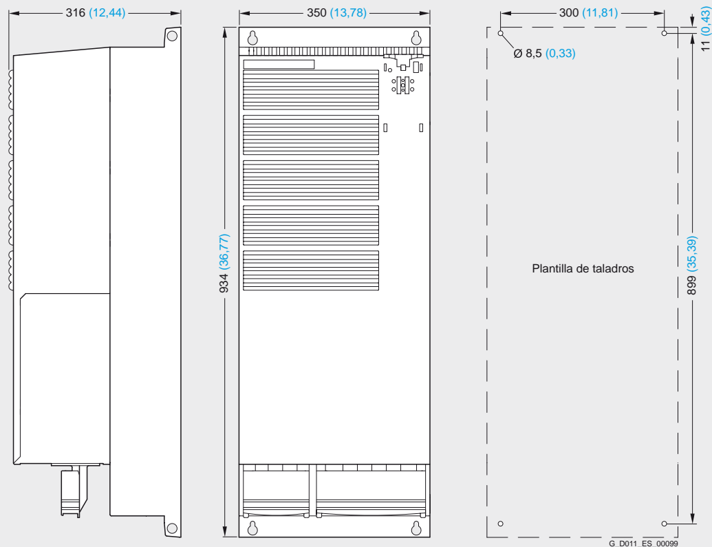
Power Module PM240 de tamaño FSF con filtro de red integrado de clase A
